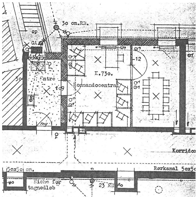
Grundtegning fra før ombygning, hvor korridoren (nederst) blev lagt til KC'en.
