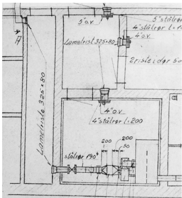
Tegning over ventilationsanlægget. Det er ikke lykkedes at identificere formålet med den lange smalle gang, som indsugningsluften passerer gennem.
