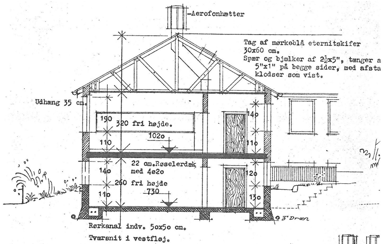
Tværsnit af bygningen.
