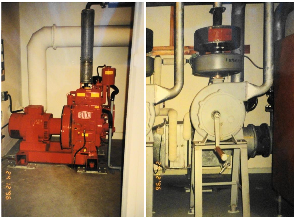
Nødgenerator og ventilationsrum i 1996. Foto udlånt af Beredskabsstyrelsen.
