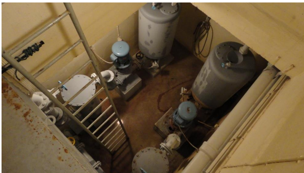
"Sump" med pumper til spildevand mv. Foto Poul Holt Pedersen.
