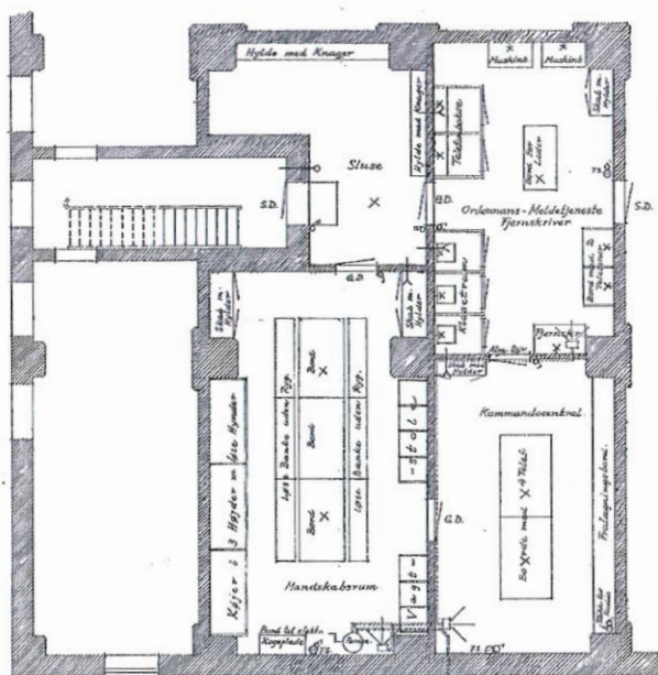
Grundplan og indretningstegning af Distriktskommandocentral nr. 5 i Glostrup 1939 med gassluse, opholdsrum til vagtmandskabet med hånddrevet ventilationsapparat, melderum med 2 telefonbokse og en fjernskriver og kommandorum. Læg mærke til de tre nødklodset rum som er opstillet i melderummet.
