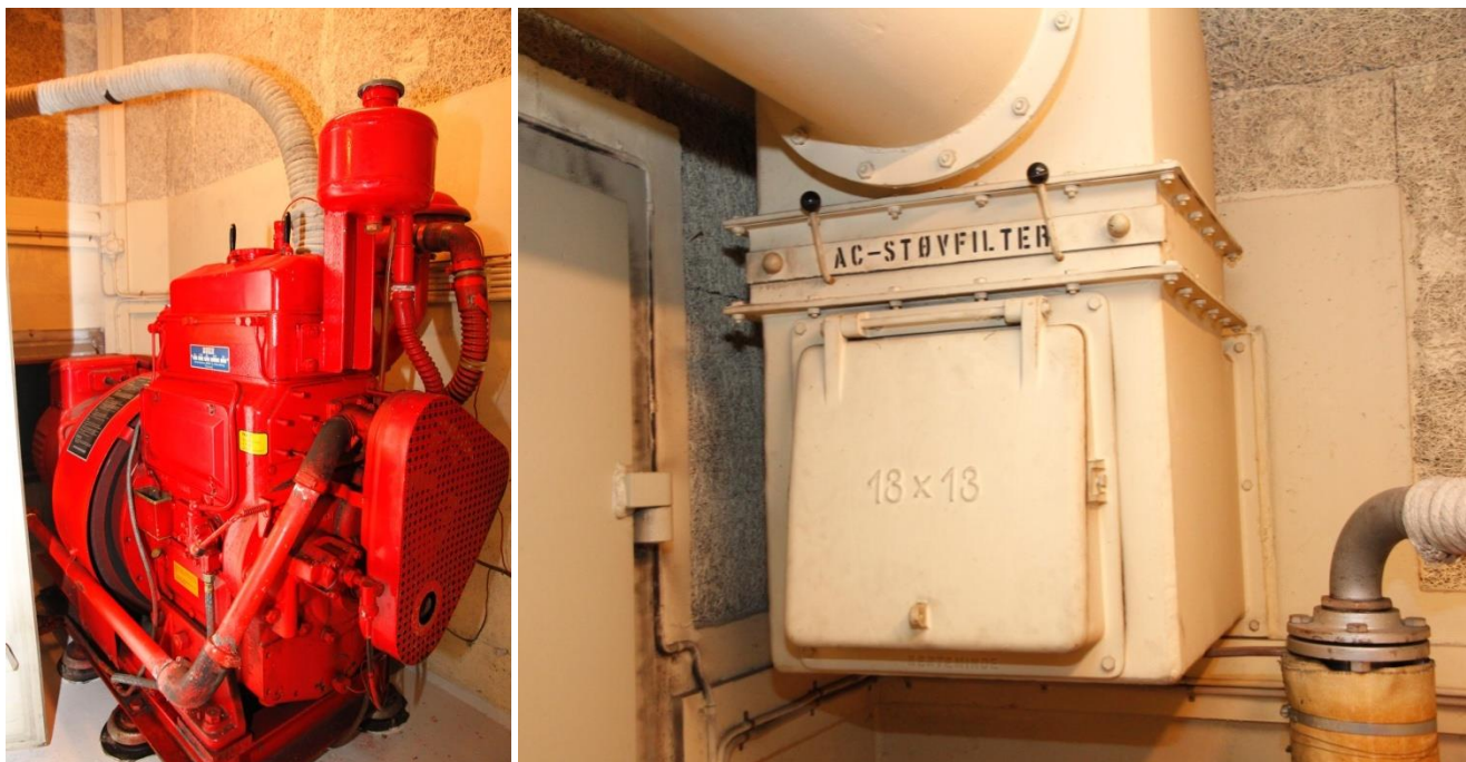
Nødgenerator (til venstre) og filter mod atomare og kemiske kampstoffer (til højre). Foto: Peter Rask 2012.
