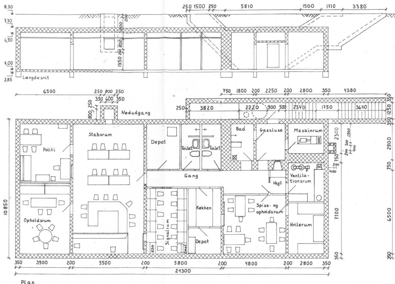
Grundtegning og tværsnit af bunkeren. Udlånt af Københavns Brandvæsen.
