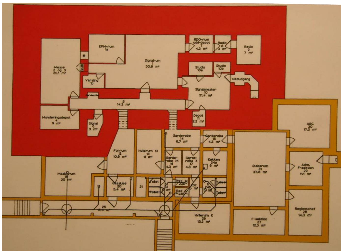
Grundtegning efter ombygning. Bunkerens samlede areal er 370 m 2 (150 for den oprindelige bunker og 220 for tilbygningen). Foto Tønnes Schrøder.
