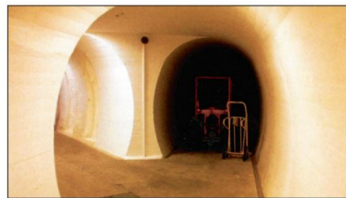
Indgangstunnelen med sidegang, der skal absorbere trykbølge.
